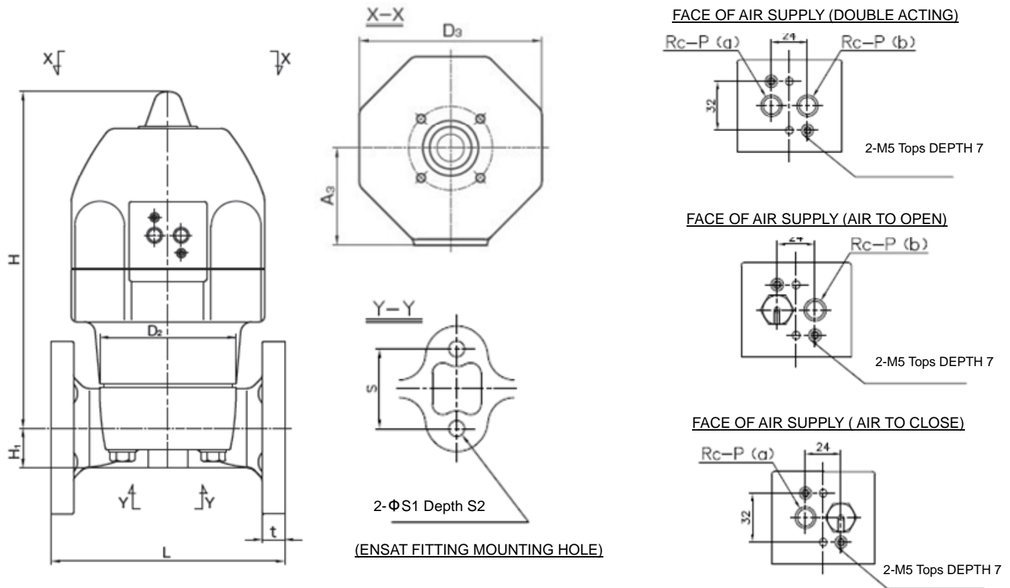
■ JIS, DIN (Unit: mm)
